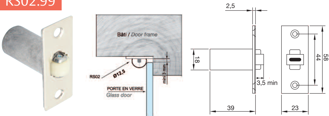
Galet avec rouleau nylon, réglable (3 à 10 mm) Blocking roller keep, adjustable (3 to 10 mm)
