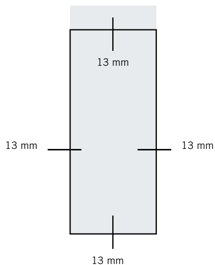
DIV - LT Anta Intelaiata con listelli trasversali - Framed panel with horizontal cross profiles - Gerahmte Tür mit Querleisten
