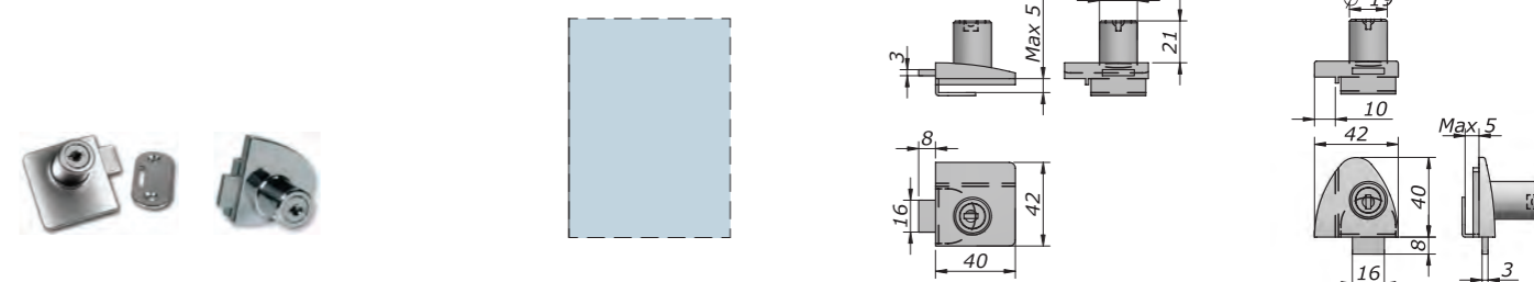
Serratura doppia senza tacca per mobili Double furniture lock without cut-out
